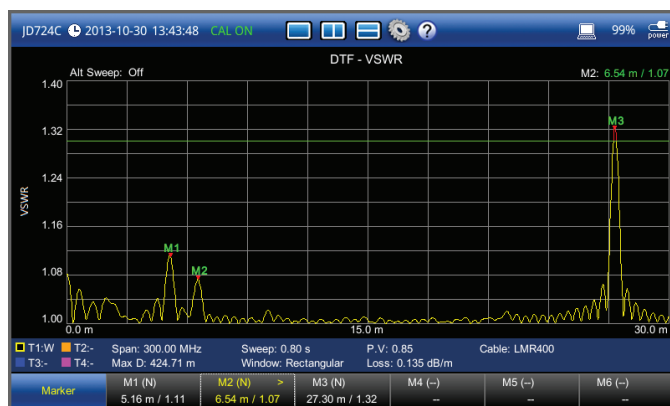
DTF — VSWR
